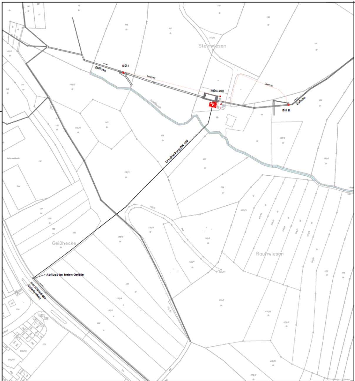
Übersichtsplan Regenüberlaufbecken der Stadt Musterstadt
