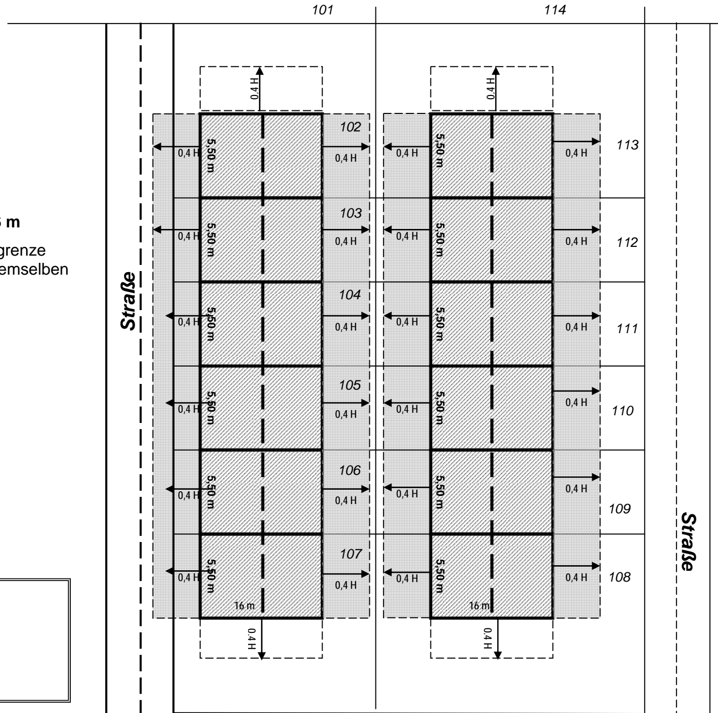
Abb.: 6.8a - Schematische Darstellung Abstandflächen bei Reihenhausbebauung
